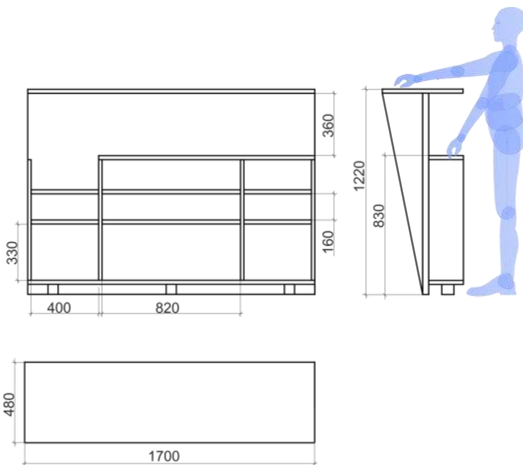
Рисунок 1 - Эргономический анализ. Касса
